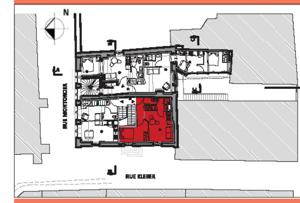
PLAN DES LOTS NIVEAU 1
