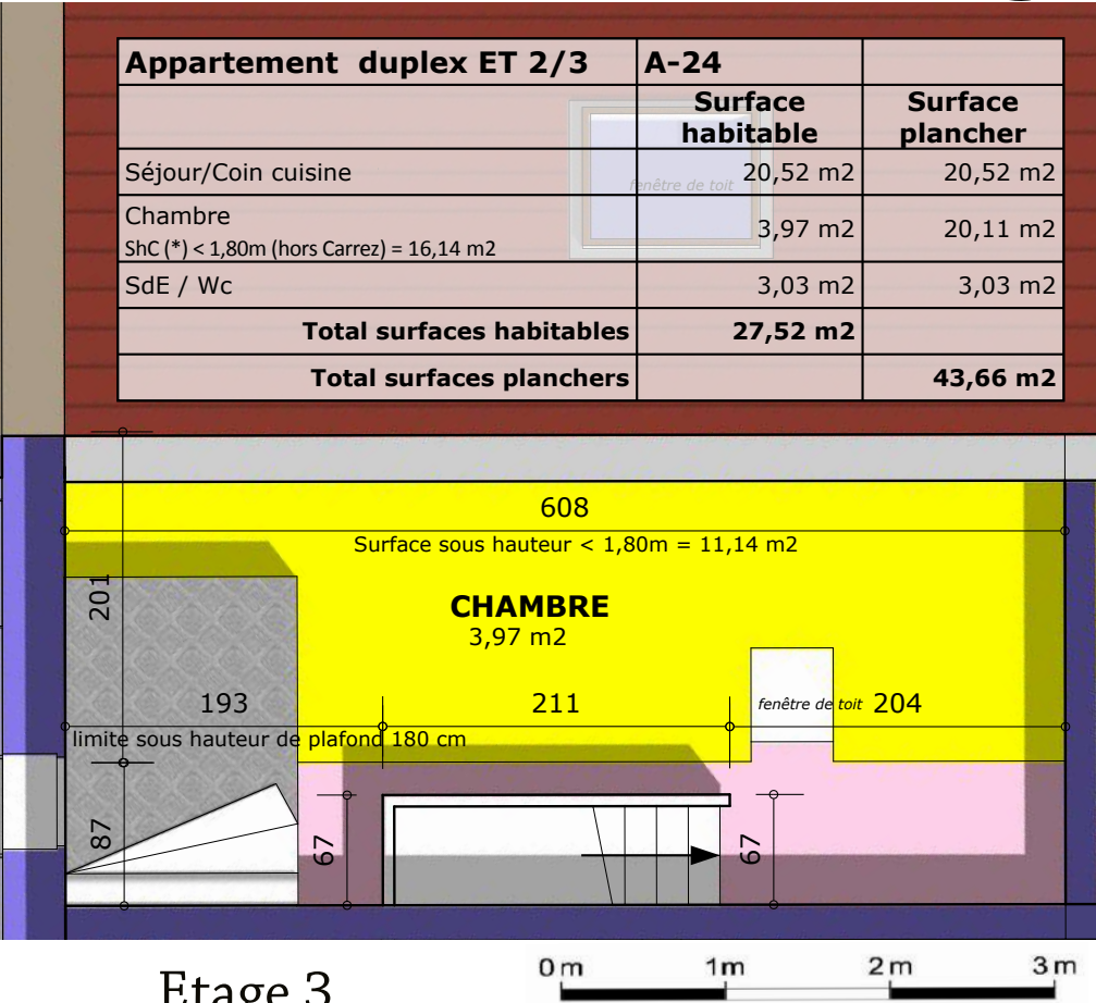
Appartement Lot n° 24 - 2 pièces 27,5 m²
