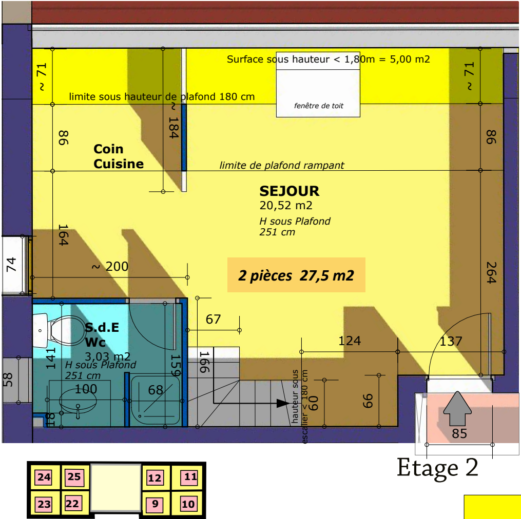
Bâtiment A - Etages 2/3 duplex
